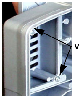
Рис. 28а - Снимите два винта V, крепящие решетку к обтекателю, и снимите решетку.
