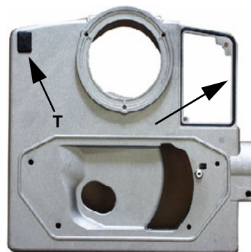
Рис. 28с - Установите поставленную прокладку в специальное гнездо в обтекателе горелки и поставьте пробку обтекателя Т.
