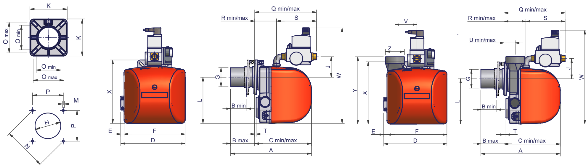
Схема сверления плиты котла
