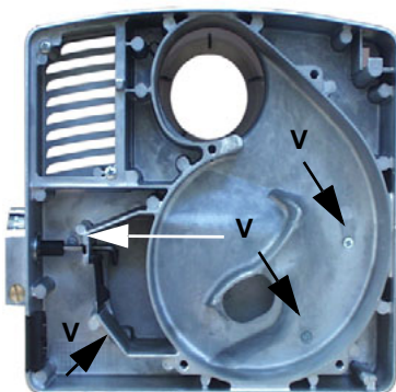
Рис. 28б - Снимите золотник, отвинчивая 4 винта V.
